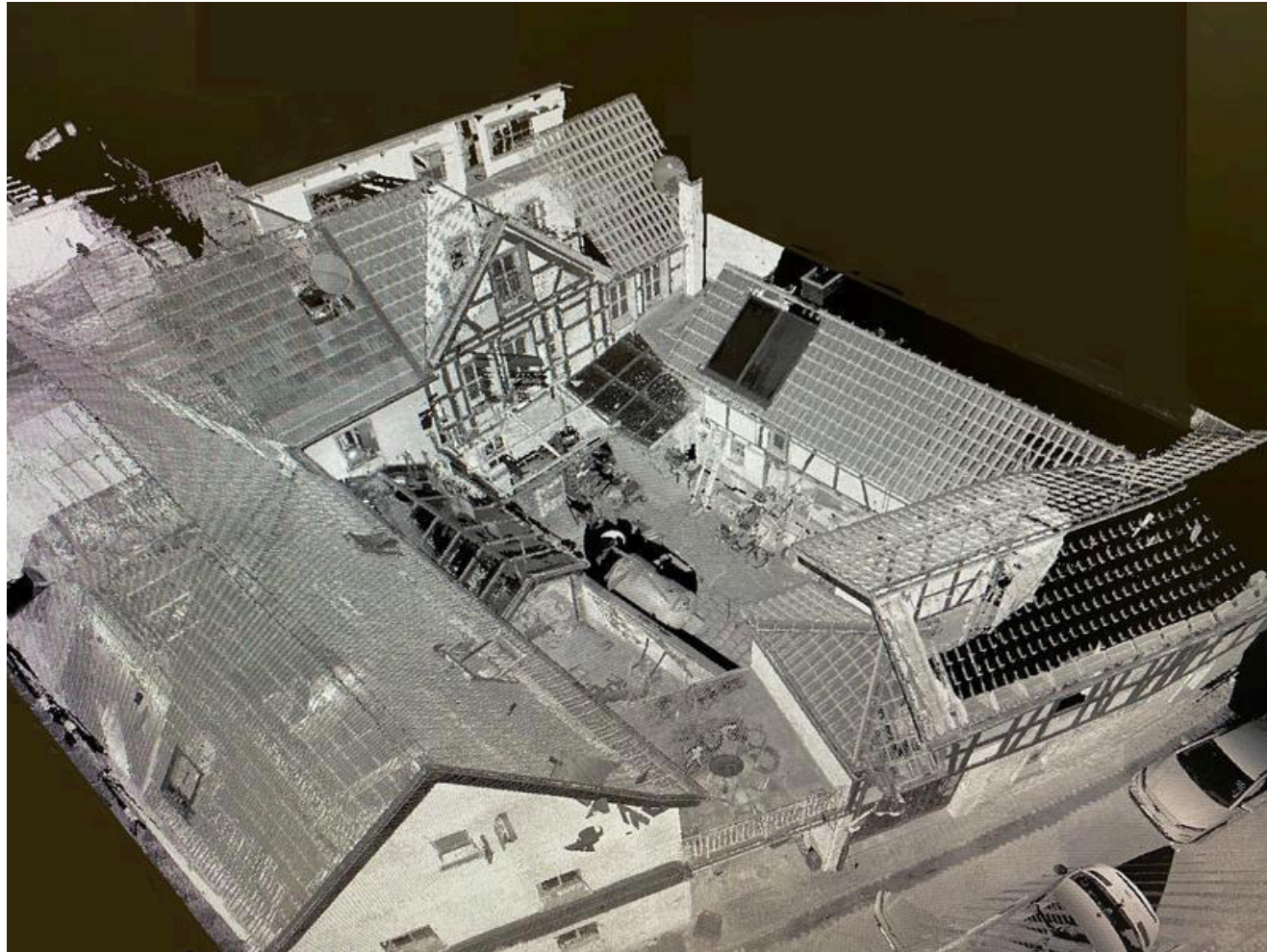
Haus Heymann Derna: Scan-Bestandsaufnahme in 2021 nach der Flut von Florian Böcker , Remscheid .
