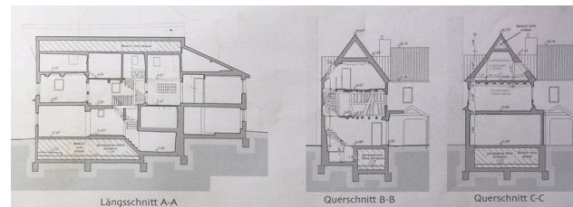
Bestandszeichnungen nach den Scan-Aufnahmen des Büro Böcker.
